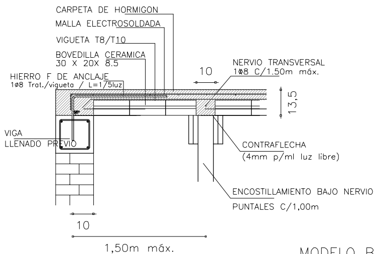
MODELO BOVEDILLA CERÁMICA
