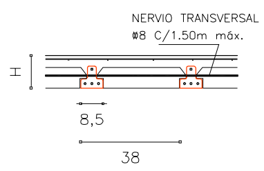
MODELO BOVEDILLA EPS
